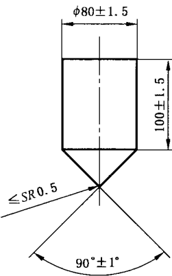
图 5 试验锥
