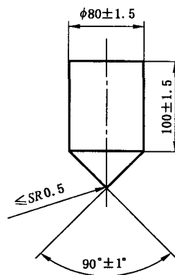
图 5 试验锥
